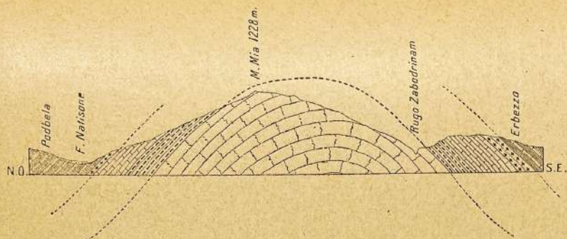
Fig. 16. — Sezione attraverso il M. Mia.
