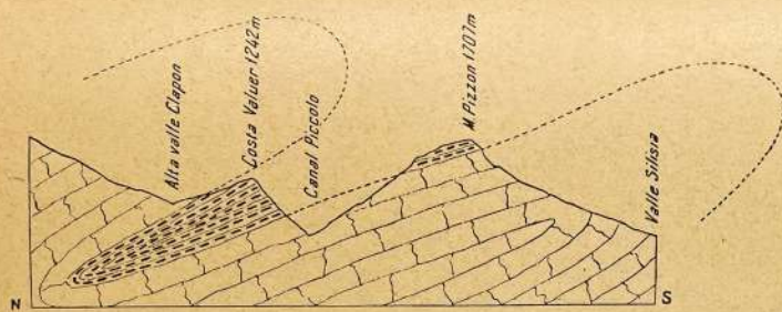
Fig. 81. — Sezione attraverso l'alto Canal Piccolo della Meduna.
