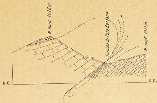
Fig. 34. — Sezione attraverso la Forcola di Pala Barsana.
