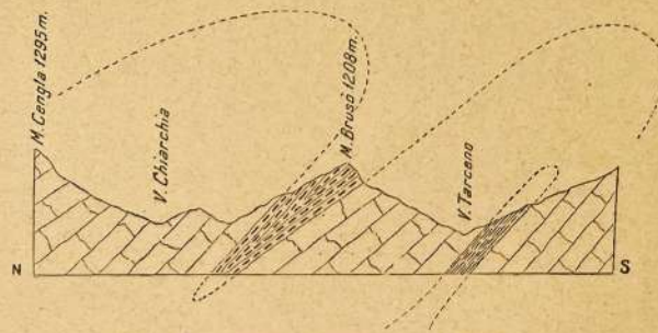
Fig. 84. — Sezione attraverso il M. Brusò.
