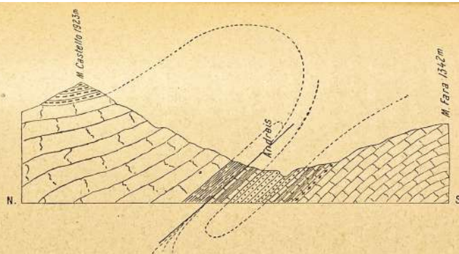
Fig. 33. — Sezione attraverso la valle del T. Alba, ad Andreis. La zona a tratti sottili e fitti, alla base della dolomia principale, rappresenta la dolomia marnosa.
