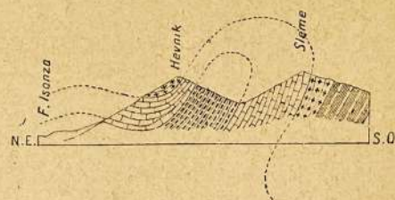
Fig. 18. — Sezione attraverso il Colovrat. (Secondo le osservazioni stratigrafiche del Kossmat).
