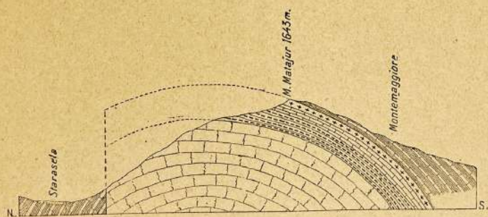
Fig. 17. — Sezione attraverso il M. Matajur.
