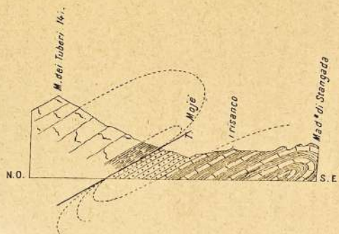
Fig. 35. — Sezione attraverso la valle del Moie, a Frisanco.
