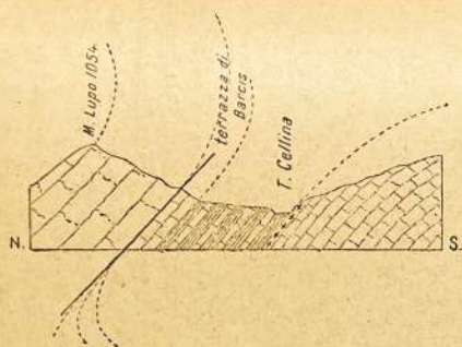
Fig. 32. — Sezione attraverso la Val Cellina a Barcis.
