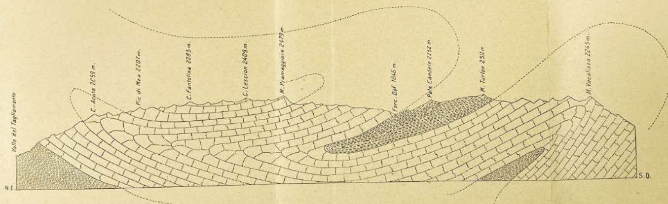
Fig. 95. — Sezione attraverso il gruppo del Pramaggiore.
