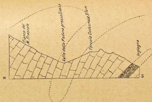
Fig. 82. — Sezione attraverso il Canal di Meduna.
