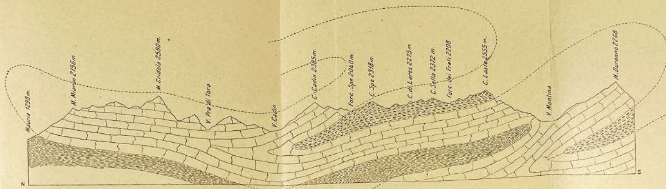
Fig. 94. — Sezione dal M. Duranno al Passo di Mauria.
