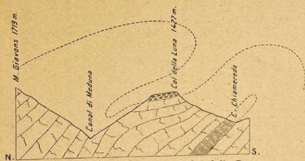
Fig. 83. — Sezione attraverso il Col della Luna.
